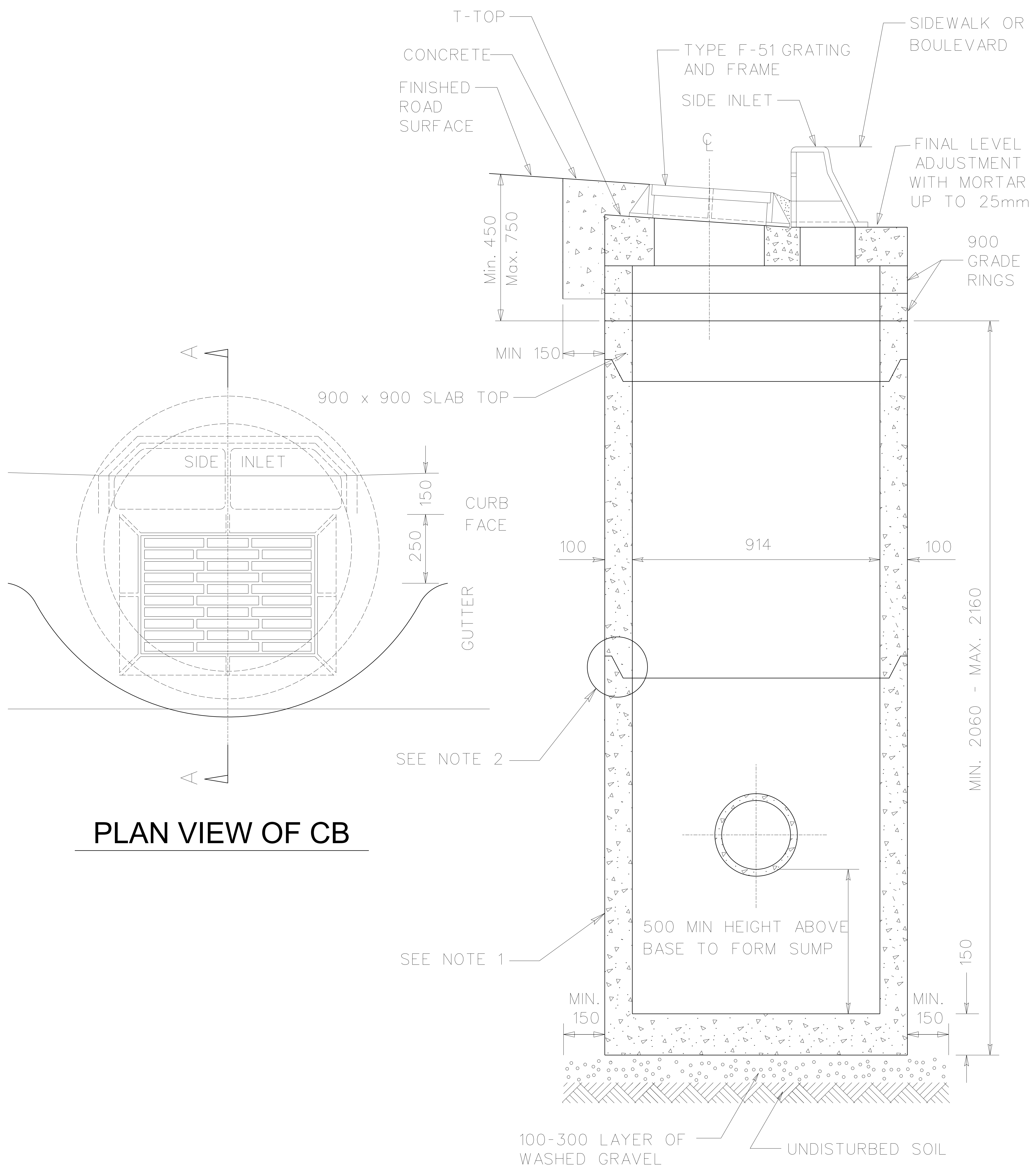
SECTION A-A
