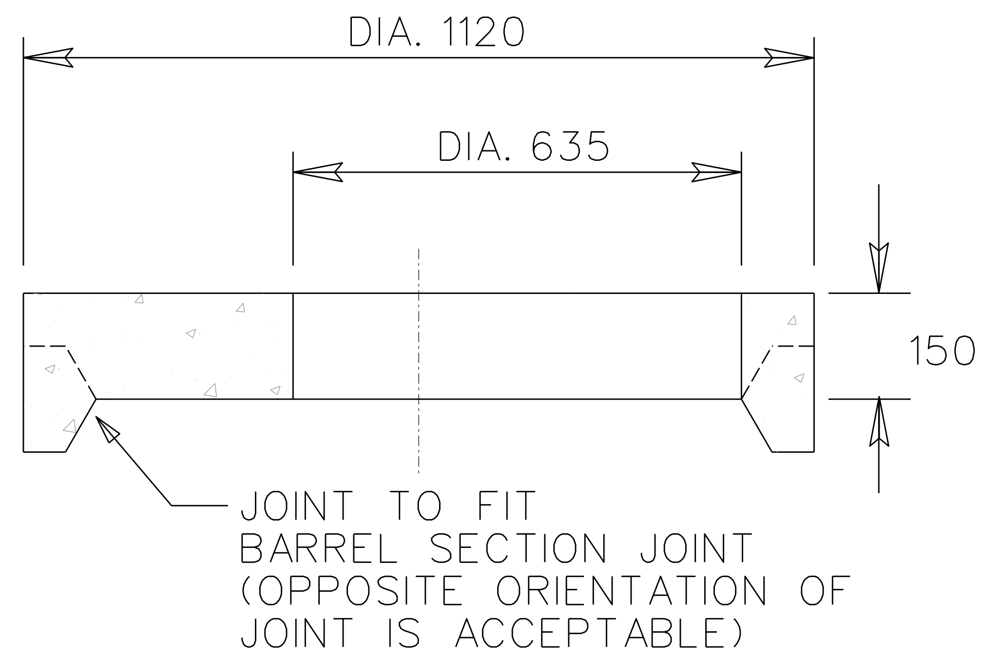
SECTION A-A
