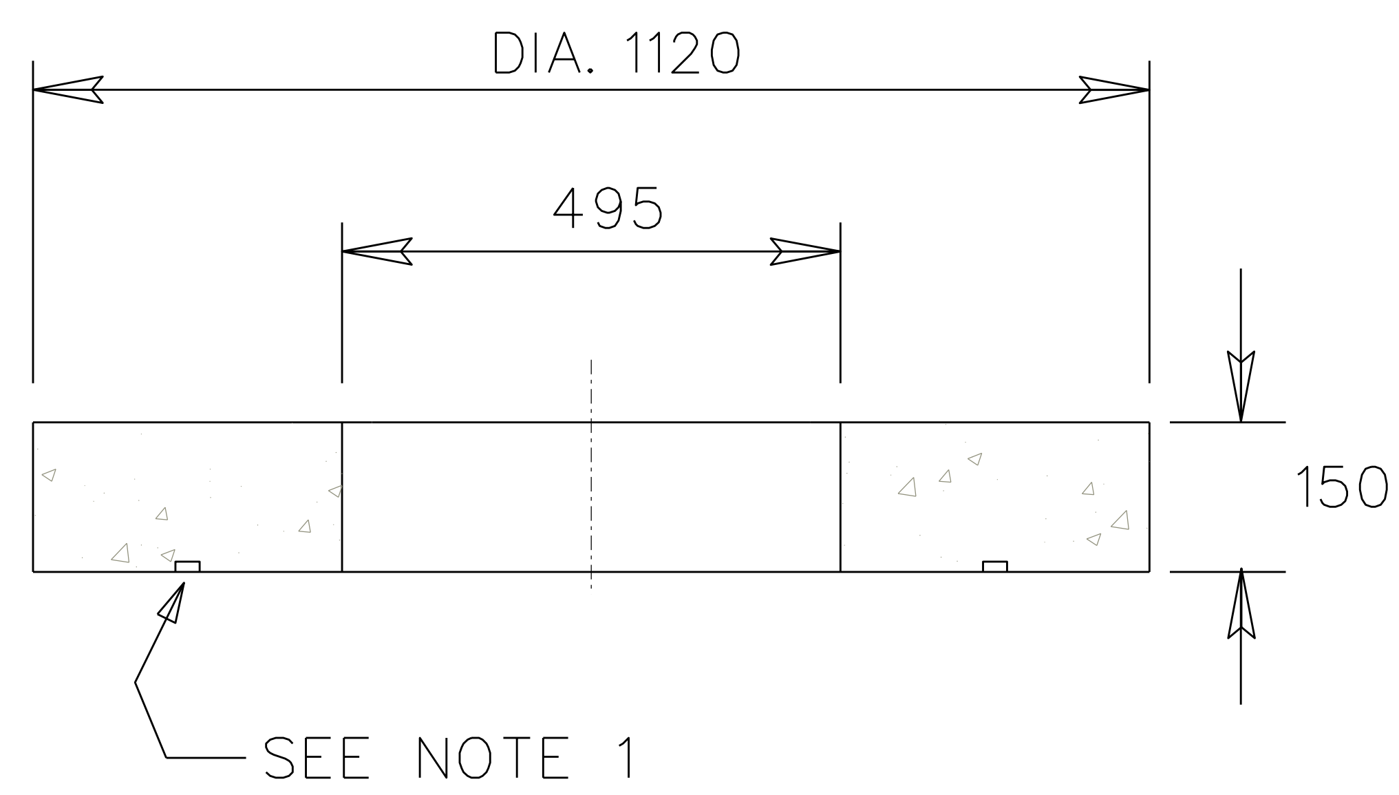
SECTION A-A
