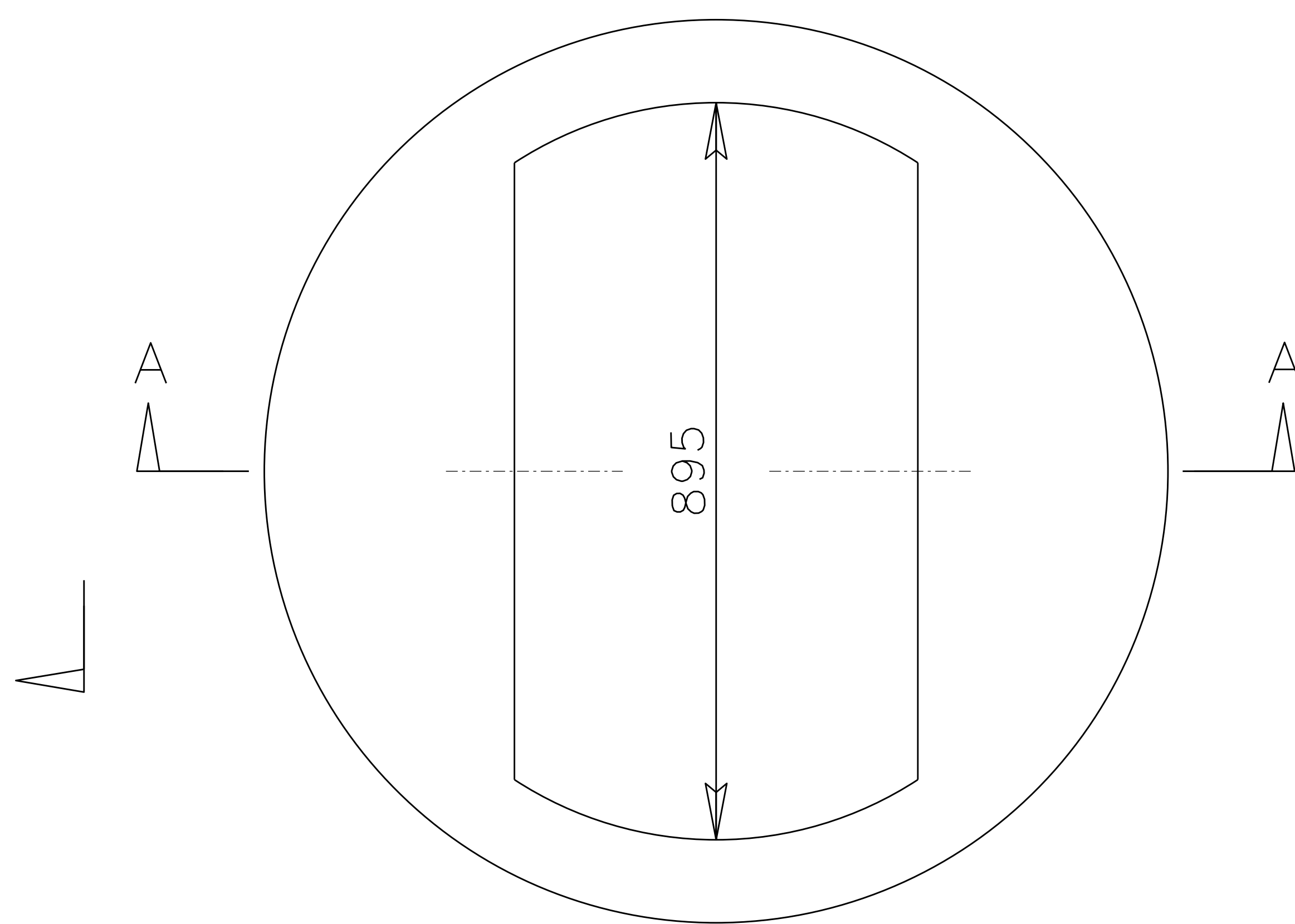
DK-7 TOP
