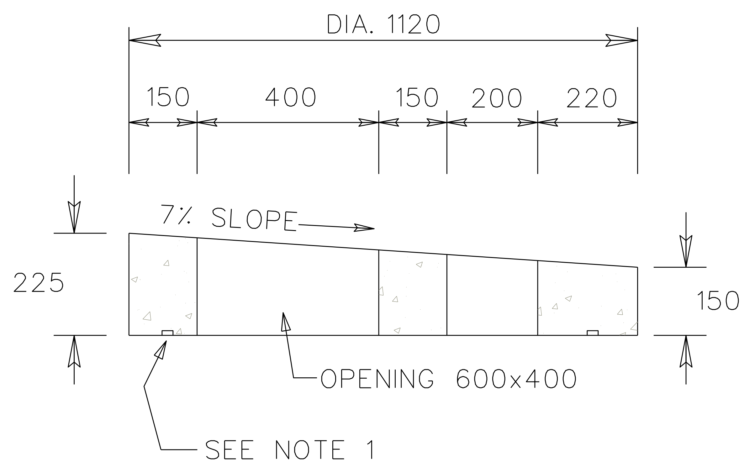
SECTION A-A
