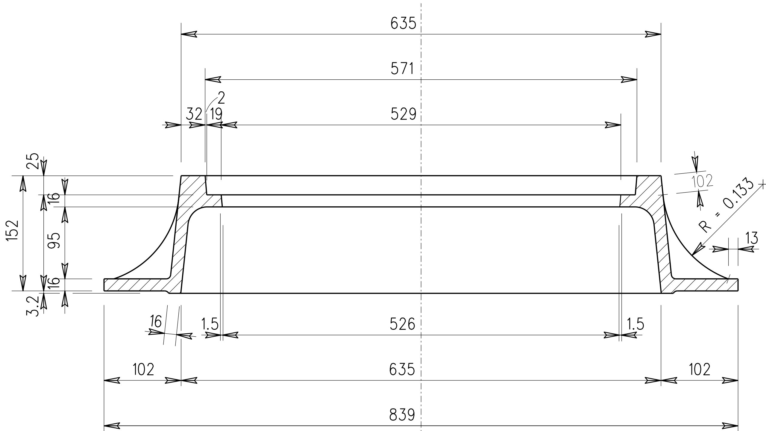
SECTION A-A
