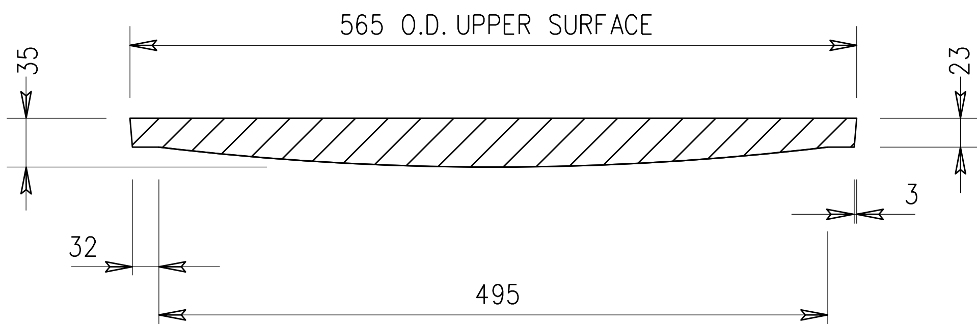
SECTION A-A
