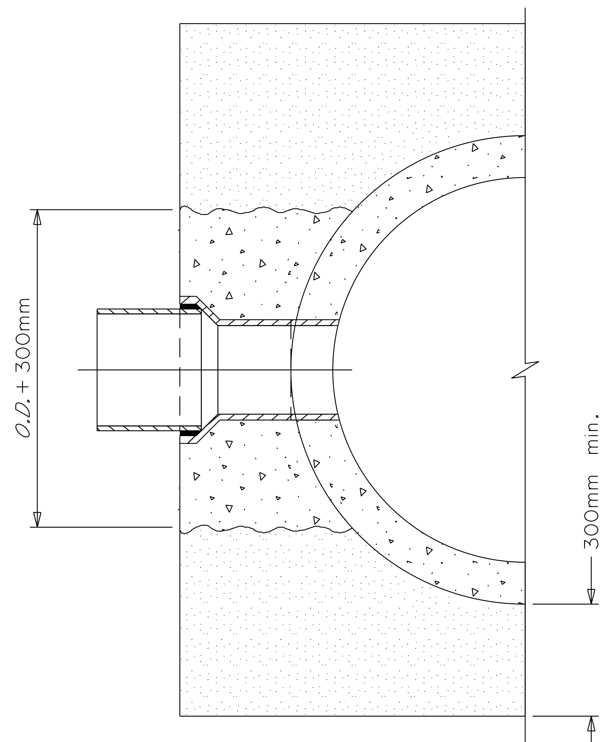
SECTION A-A
