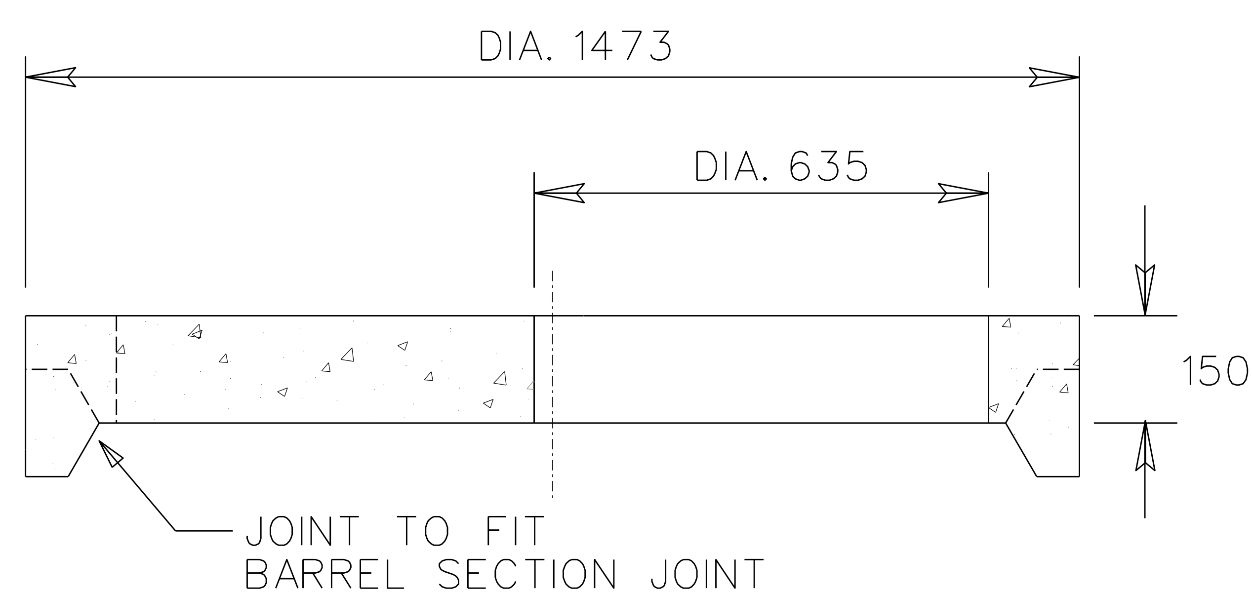
SECTION A-A
