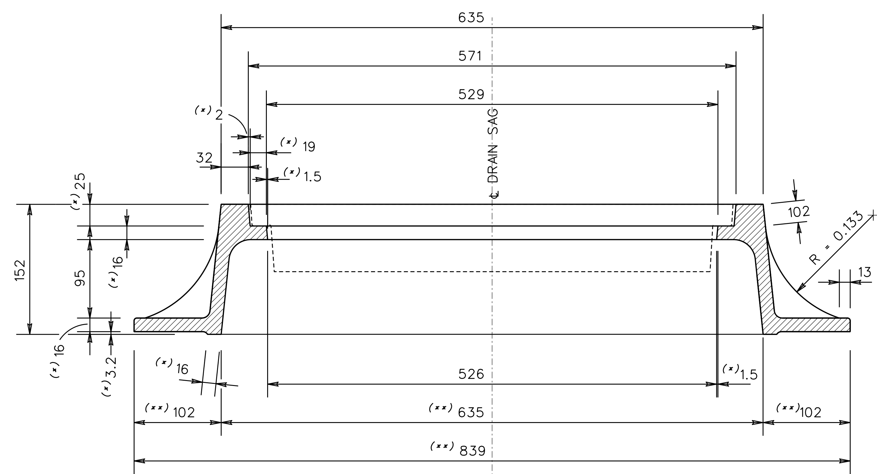
SECTION A-A
