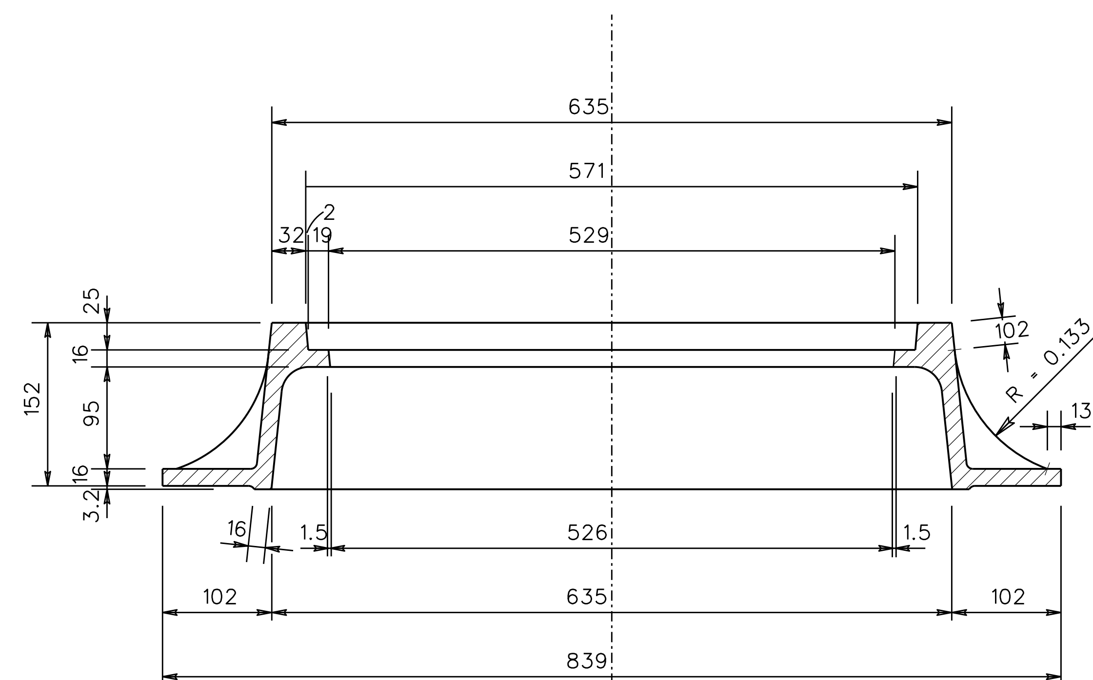
SECTION A-A
