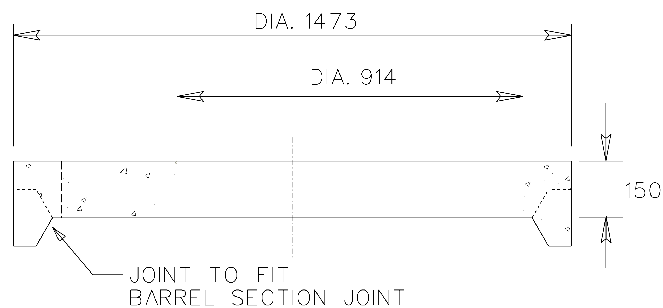
SECTION A-A
